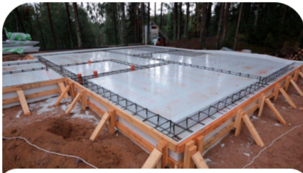
Заливка фундамента, марка М250–М300
